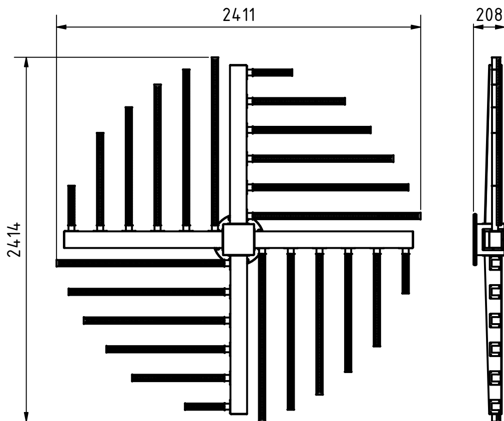
NDV-2600 ДРС Ф2600 1 шт. на проект
