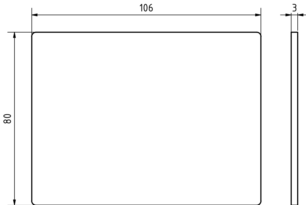
NDV-2104 Заглушка коллектора, s=3.0 1 шт. на NDV-2000; 4 шт. на проект
