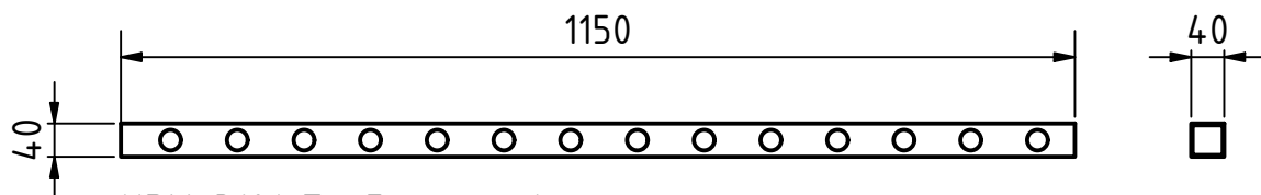
NDV-3101 Труба луча 1
