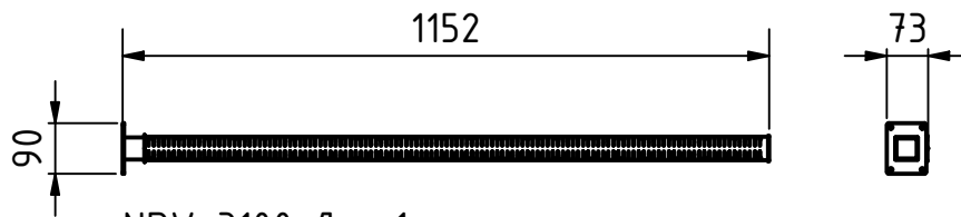
NDV-3100 Луч 1 4 шт. на проект
